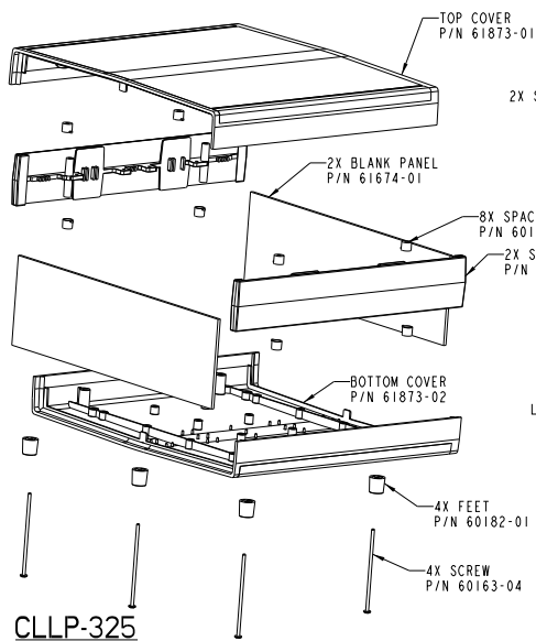
CLLP-325
